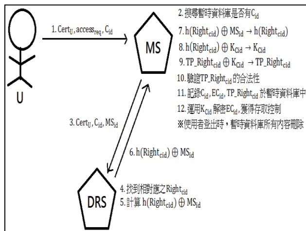
圖 2-4 使用階段示意圖
