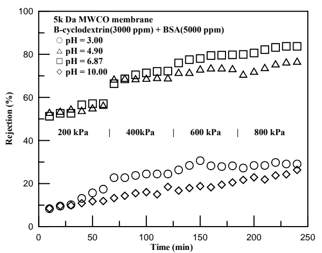
圖 8 雙溶質系統不同 pH 值下 \beta -cyclodextrin 之阻隔率變化
