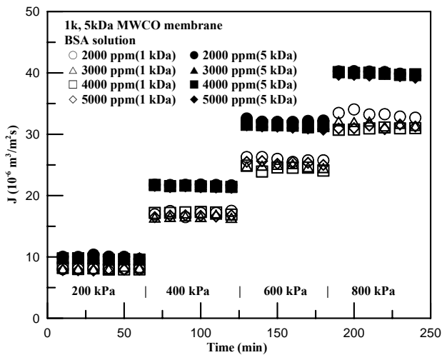
圖 4 不同 BSA 濃度下之濾速變化
