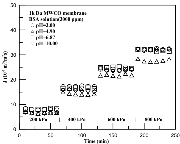
圖 5 不同 pH 值下 BSA 溶液之濾速變化
