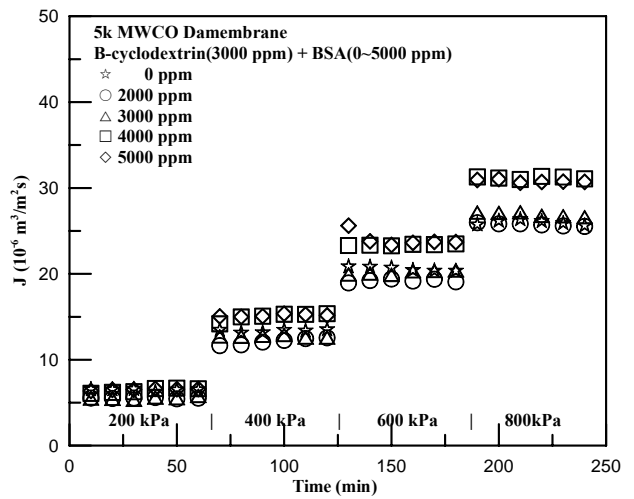
圖 6 雙溶質系統改變 BSA 濃度之濾速變化
