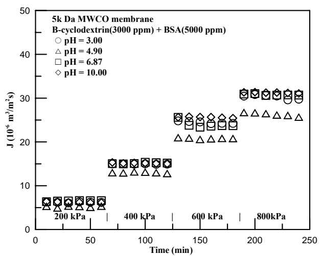
圖 7 雙溶質系統改變 pH 值之濾速變化
